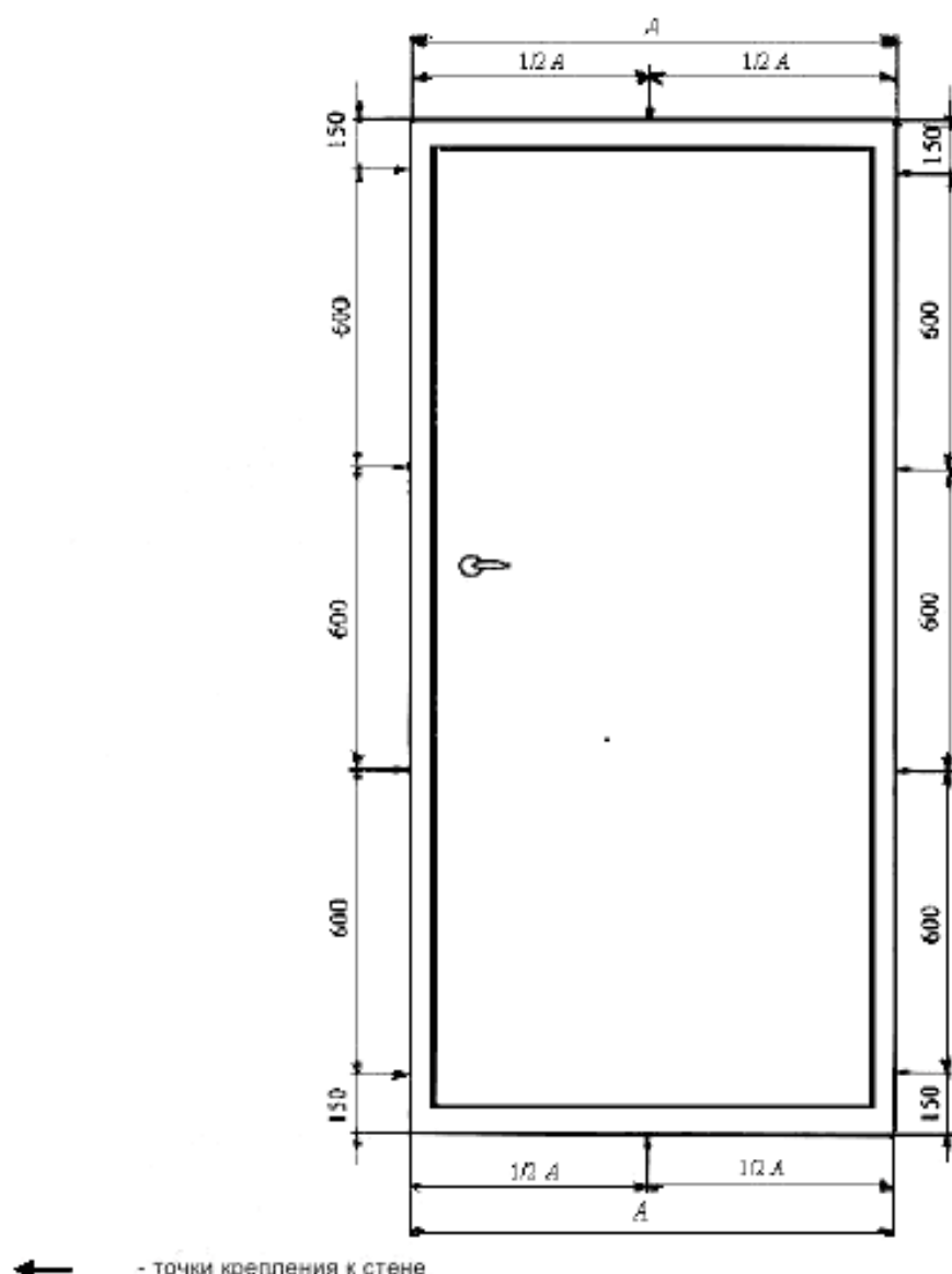
Рисунок А.1 – Пример расположения крепежных деталей при монтаже дверного блока с замкнутой коробкой
